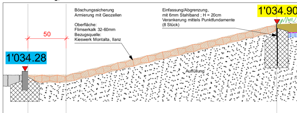
Schnitt Böschung, M 1:20
